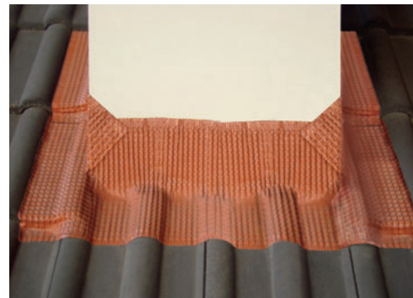
Raccordement d'un conduit de fumée
